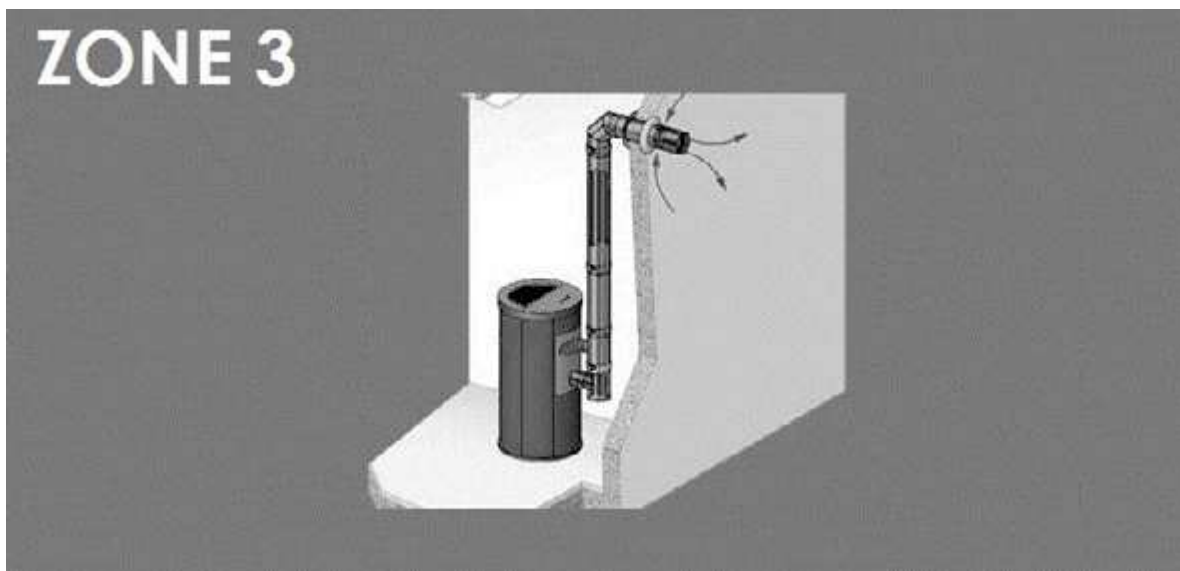
Fig. 18 - Schéma de principe du système concentrique avec terminal horizontal (ZONE 3)
