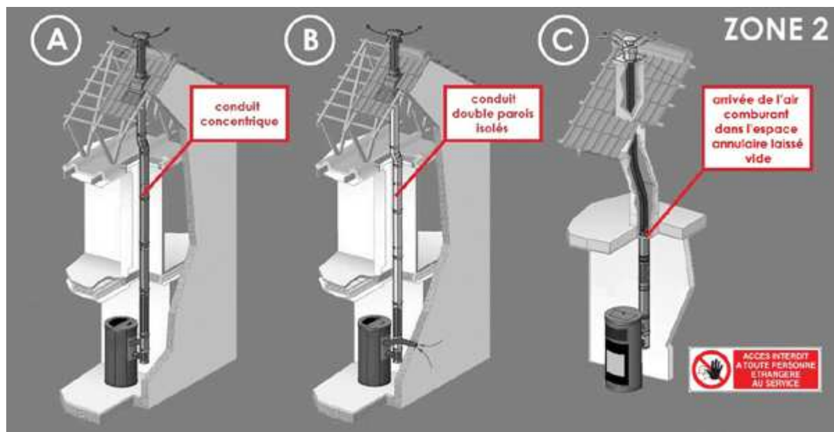
Fig. 17 - Schéma de principe des 3 types de système concentrique avec terminal vertical (ZONE 2)
