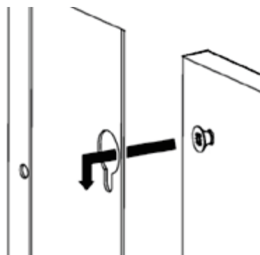
Fig. 34 - Détail de l'accrochage
