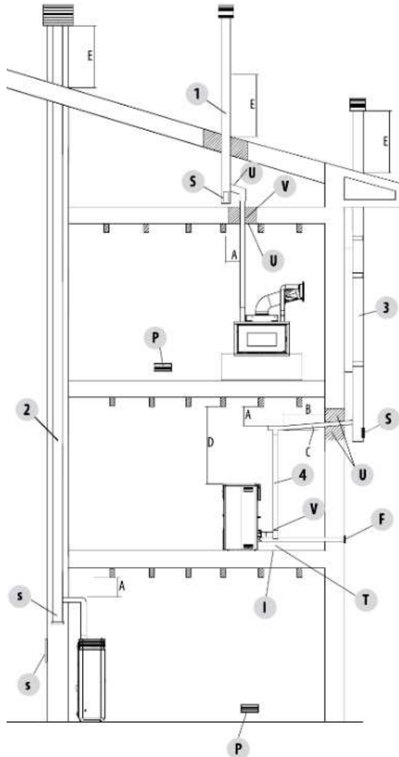
Fig. 12 - Conduit des fumées
