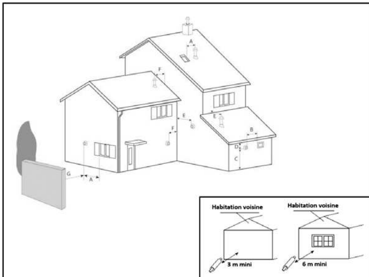
Fig. 14 - Position des terminaux
