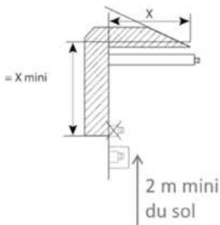
Fig. 15 - Rebord de toit
