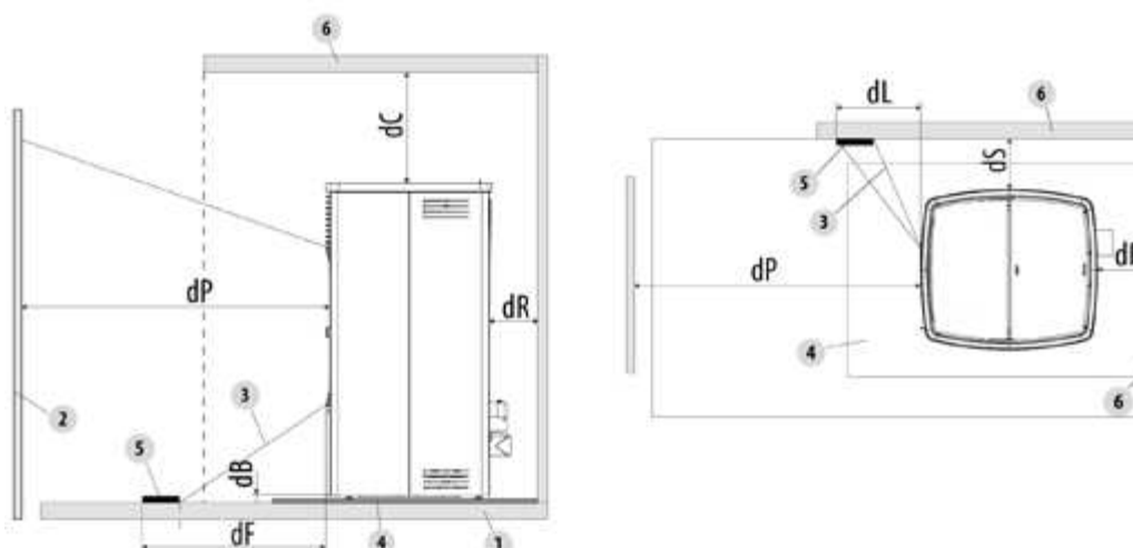
Fig. 21 - Distances de sécurité
