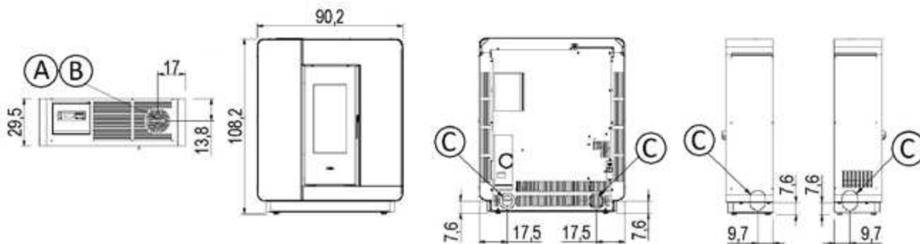
Fig. 25 - Elle Plus 7/9 UP-TWIN
