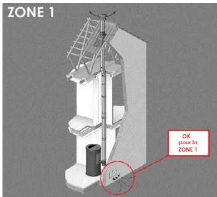
Fig. 16 - Installation possible pour tous les poêles (ZONE 1)
