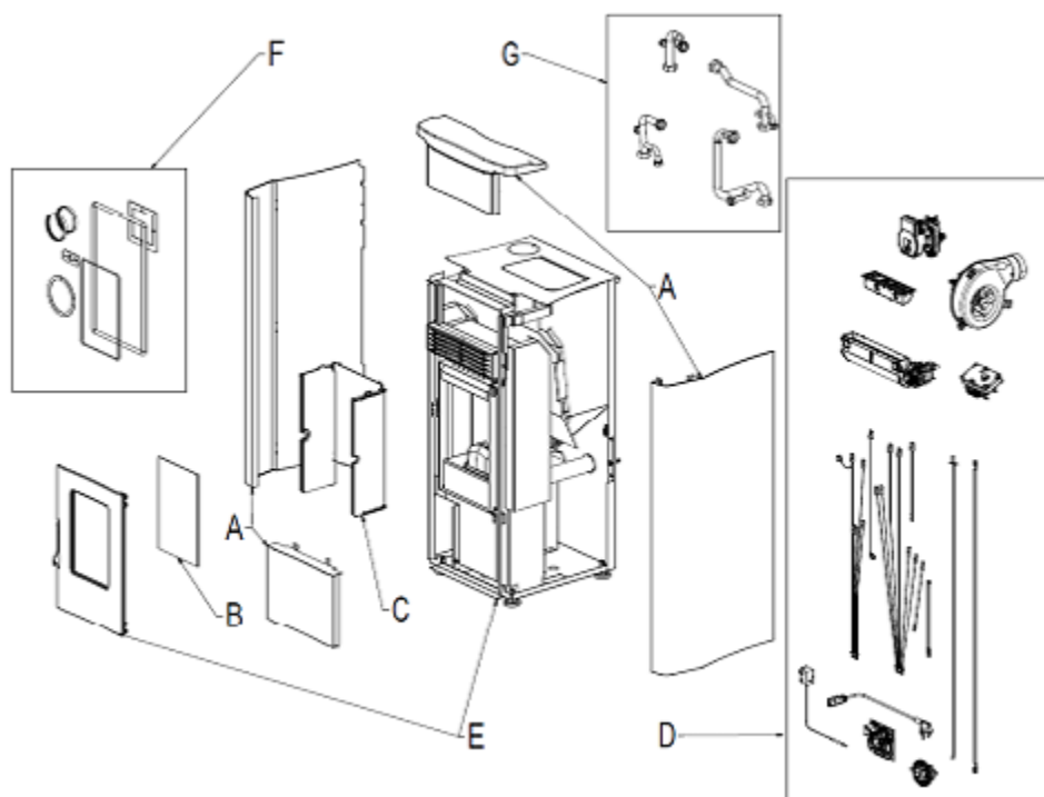
Fig. 1 - Dessin éclaté
