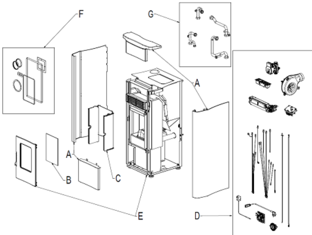
Fig. 1 - Dessin éclaté
