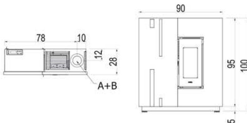
Fig. 31 - BAGGY 7 UP-TWIN T2
