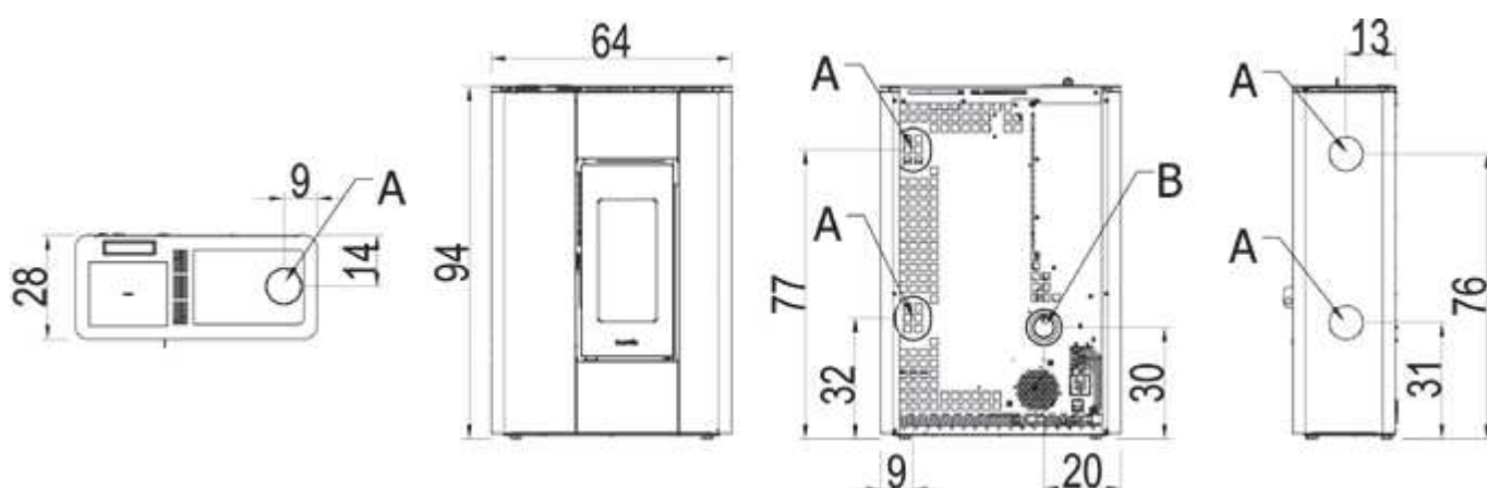
Fig. 25 - ATRIUM 5 T2 ATRIUM 5 UP ATRIUM AIRTIGHT
