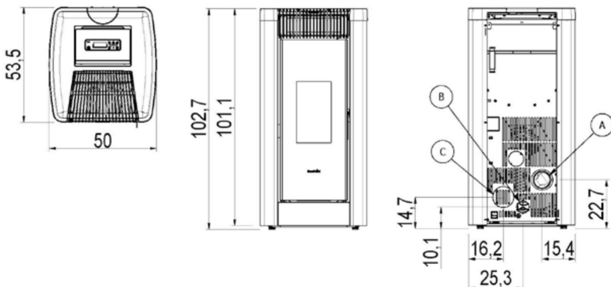
Fig. 29 - Dimensions générales: Steel 9
