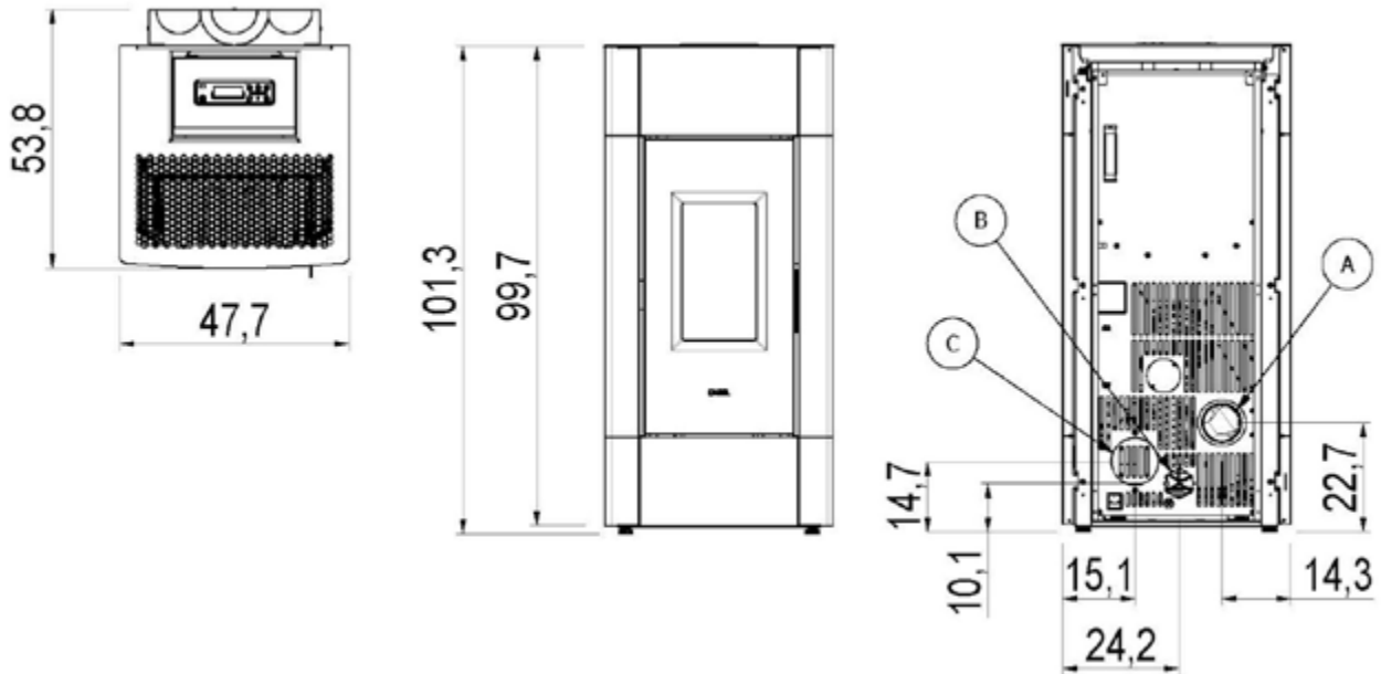
Fig. 25 - Dimensions générales: Cristal Plus 9
