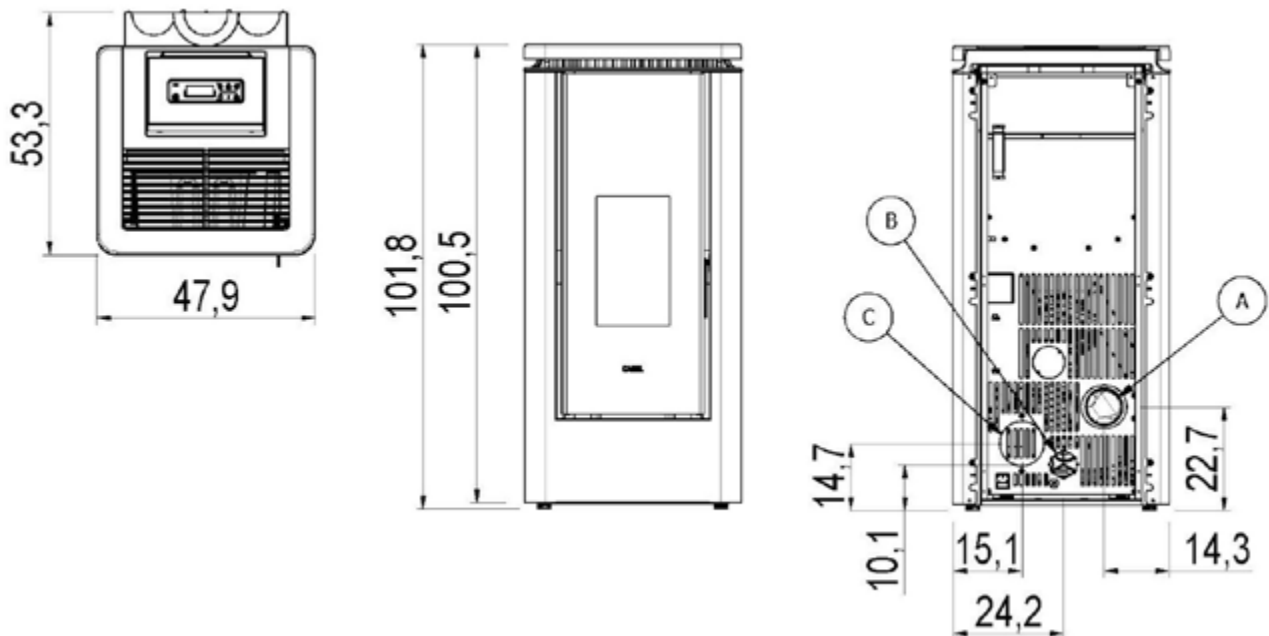
Fig. 26 - Dimensions générales: Icon Plus 9
