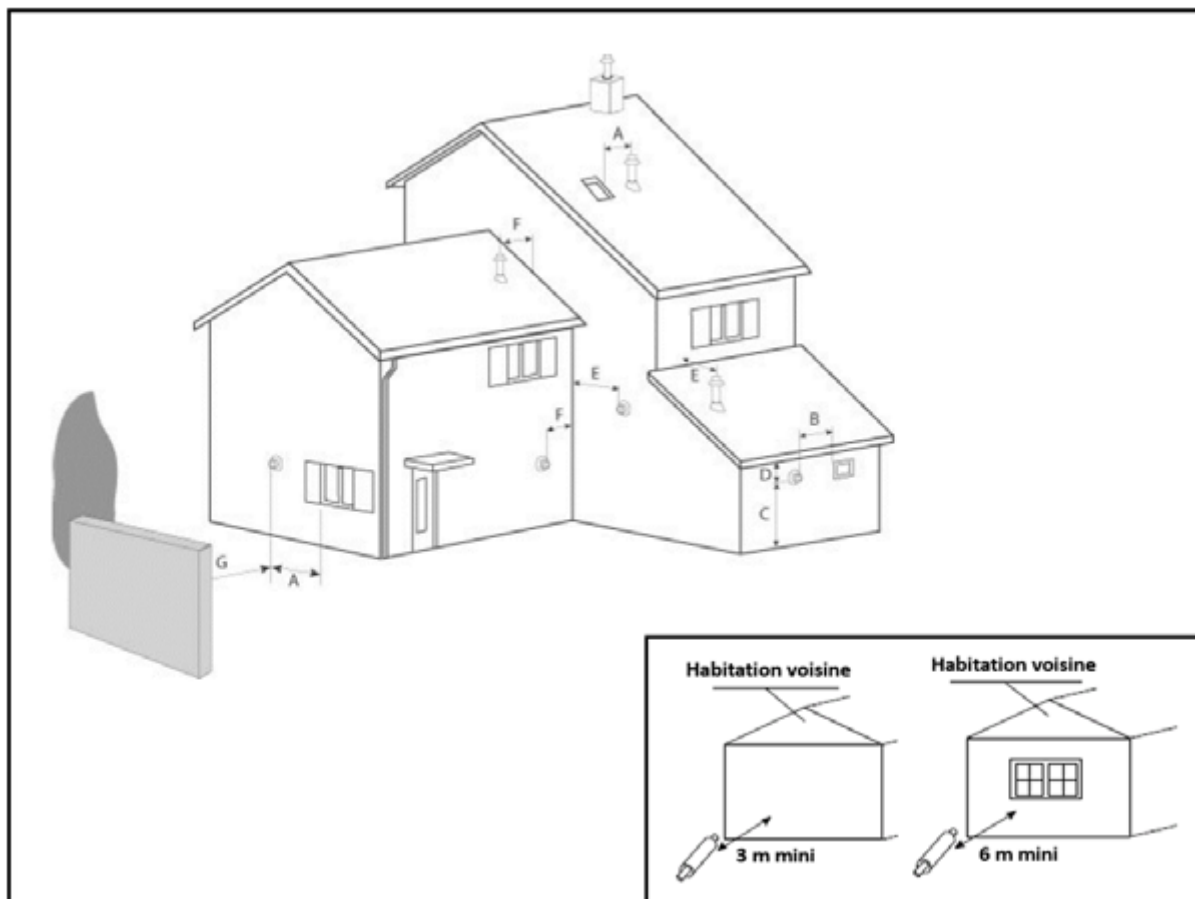
Fig. 16 - Position des terminaux
