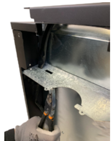
Fig. 77 - Rabattre les ailettes
