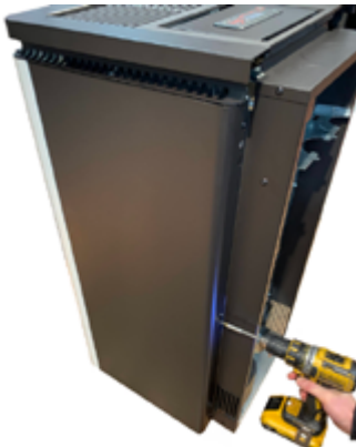
Fig. 40 - Retirer les vis postérieures
