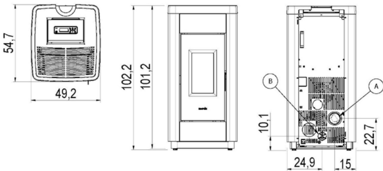
Fig. 28 - Dimensions générales: Life 9
