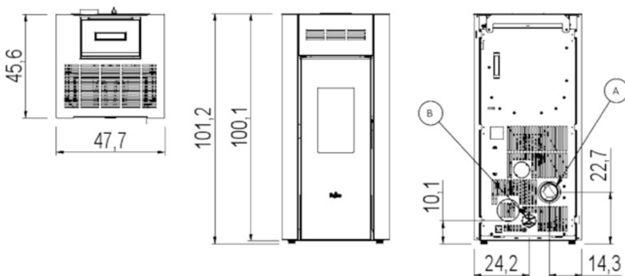
Fig. 30 - Dimensions générales: Elane 9
