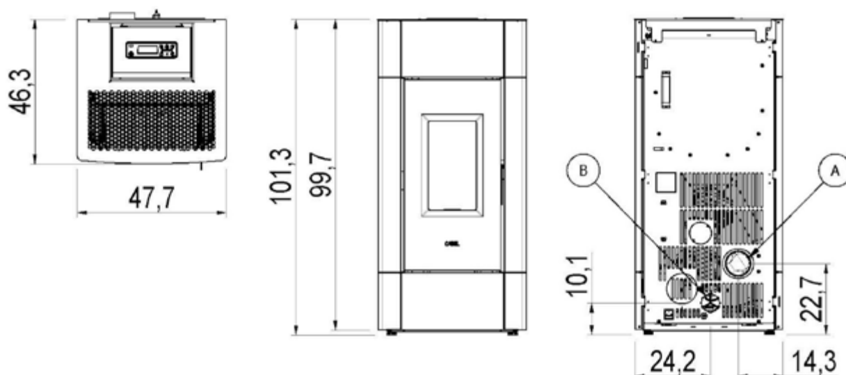
Fig. 24 - Dimensions générales: Cristal 9
