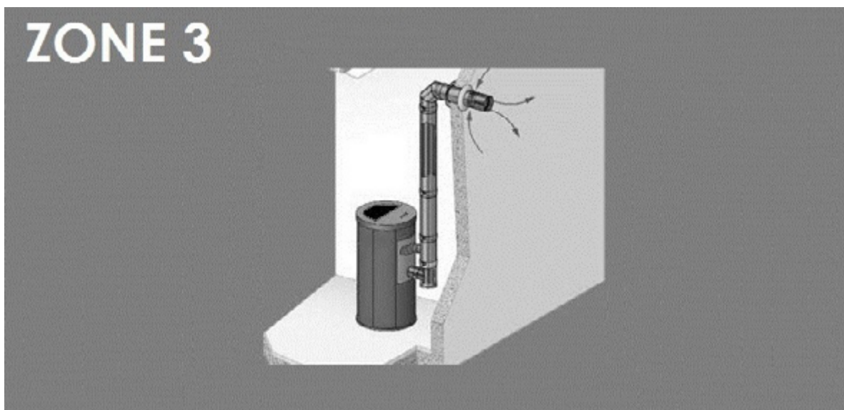
Fig. 20 - Schéma de principe du système concentrique avec terminal horizontal (ZONE 3)
