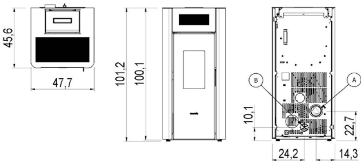
Fig. 27 - Dimensions générales: Amaranto 9
