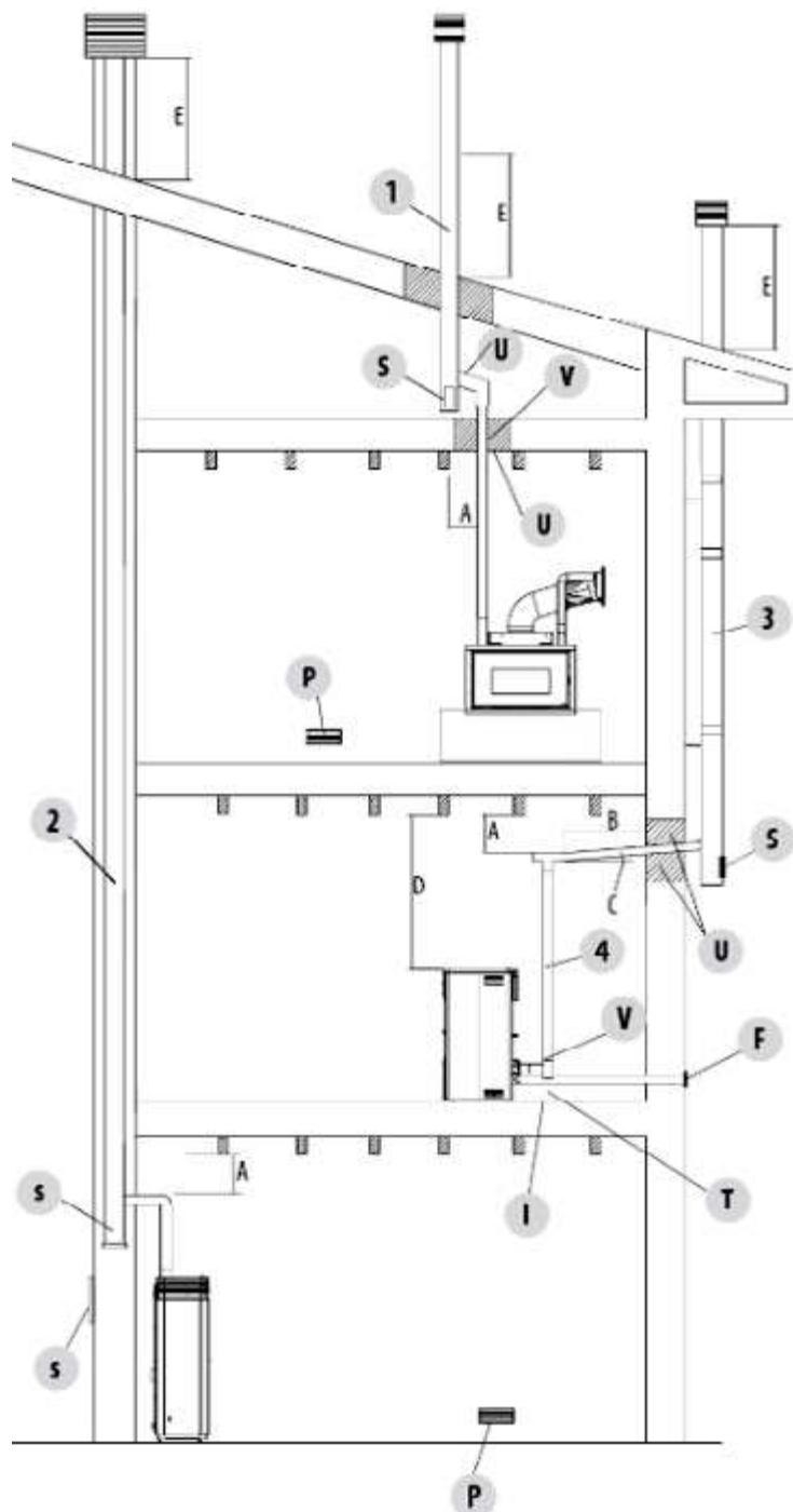
Fig. 20 - Conduit des fumées
