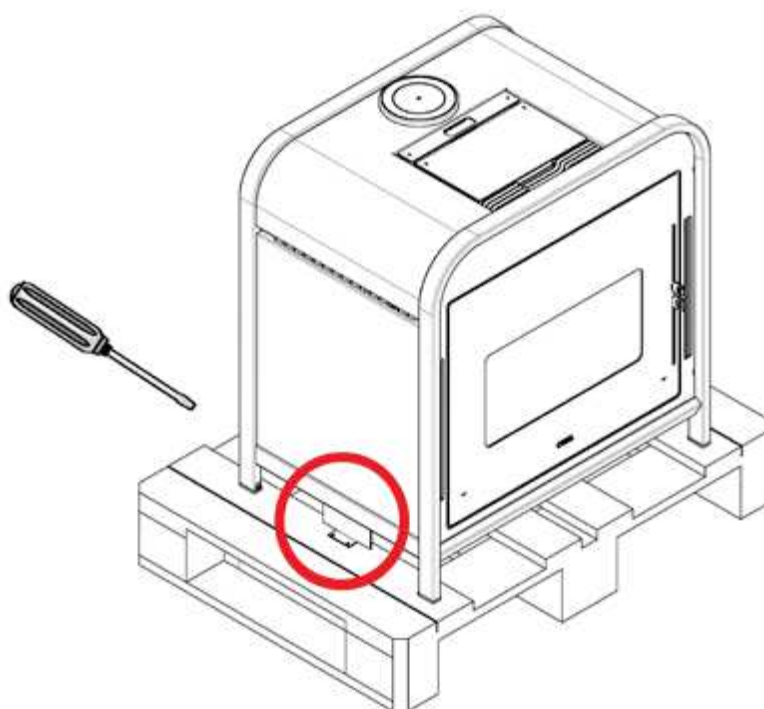
Fig. 1 - Retrait des vis + étriers
