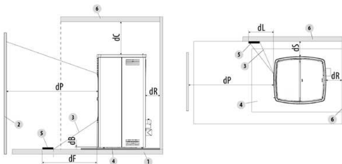
Fig. 21 - Distances de sécurité
