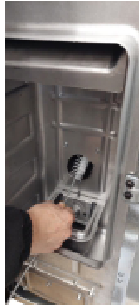
Fig. 20 - Nettoyage avec nettoie-pipes
