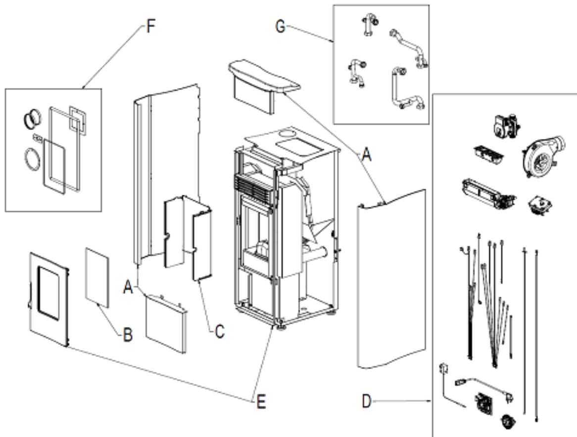
Fig. 1 - Dessin éclaté
