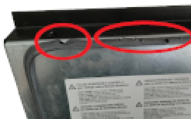
Fig. 10 - joint détérioré
