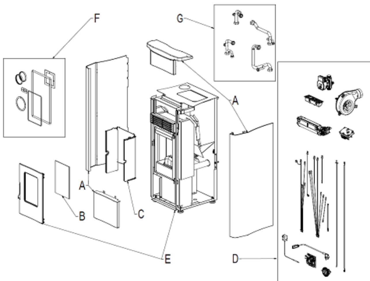
Fig. 1 - Dessin éclaté
