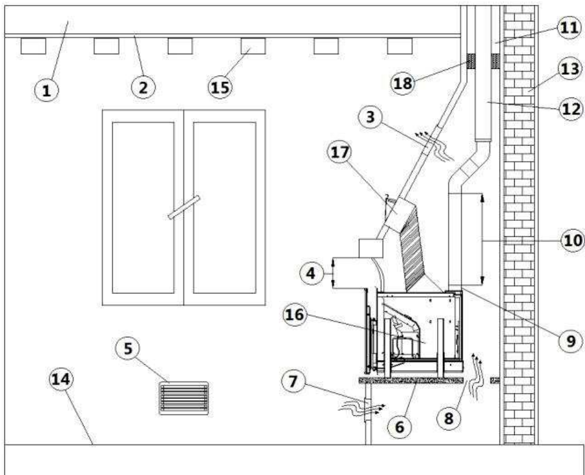
Fig. 35 - Installation sur la cheminée existante
