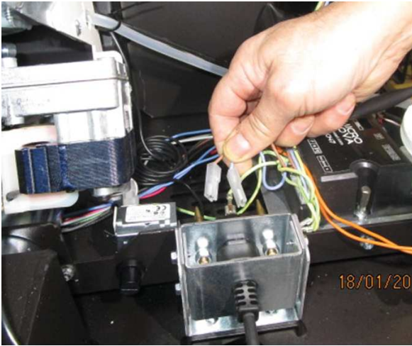
Fig. 97 - Déconnexion connecteurs type faston (bleu - marron)
