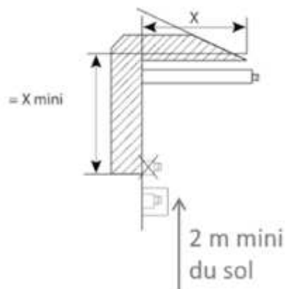
Fig. 16 - Rebord de toit
