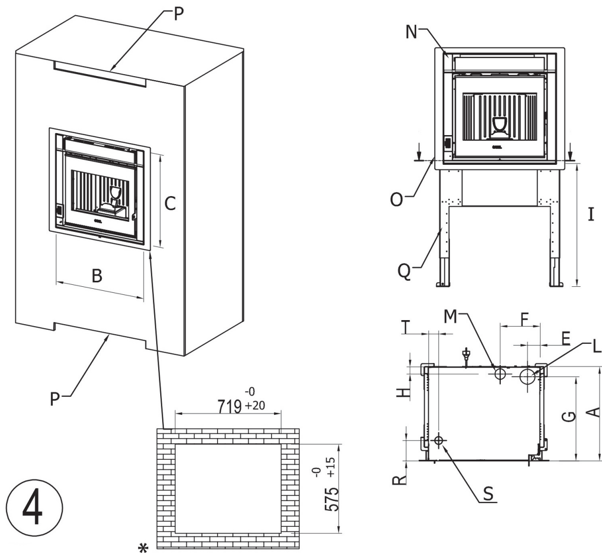
Fig. 26 - ZEFIRO-ZEN tiroir + cadre
