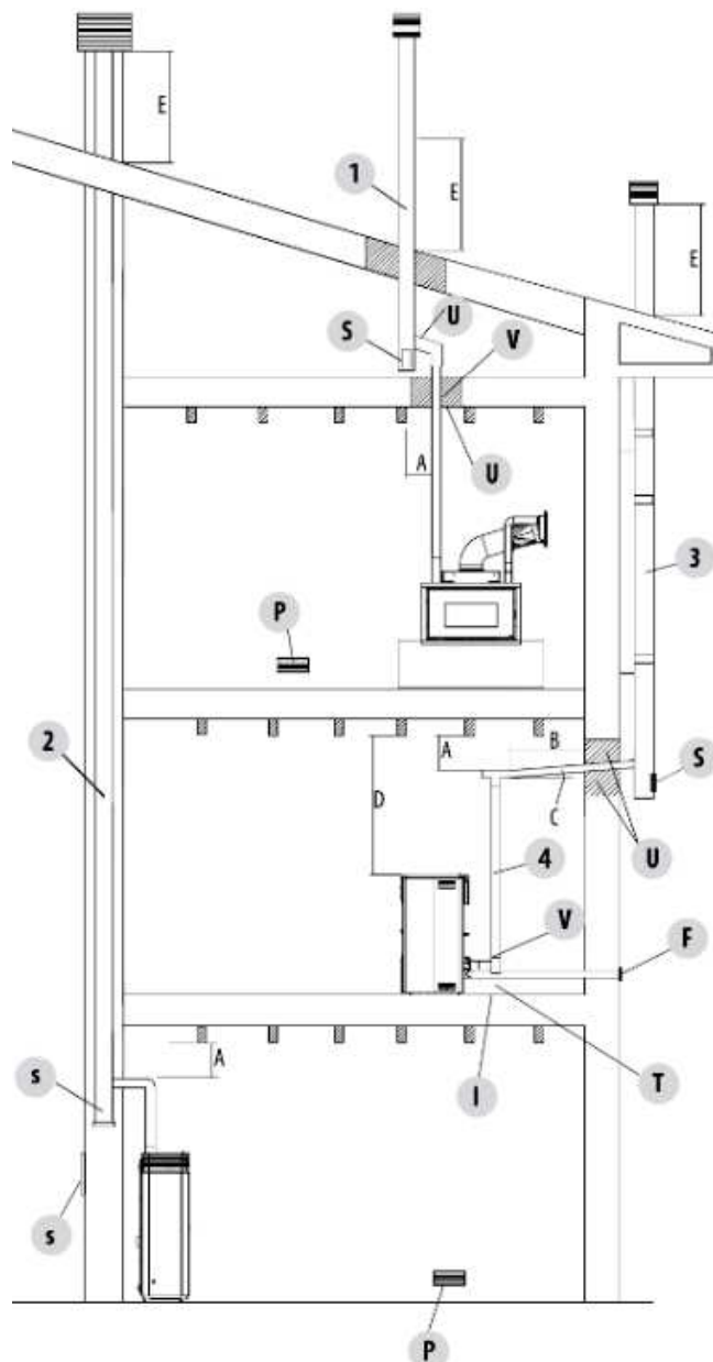
Fig. 13 - Conduit des fumées
