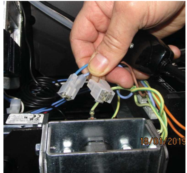
Fig. 98 - Connexion connecteurs type faston doubles
