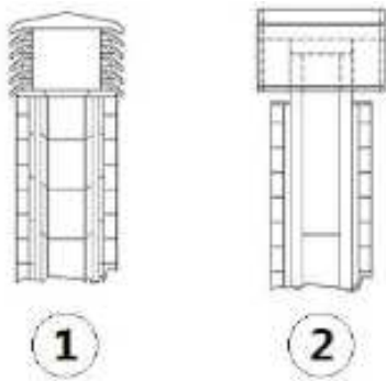
Fig. 6 - Sortie de toit coupe-vent
