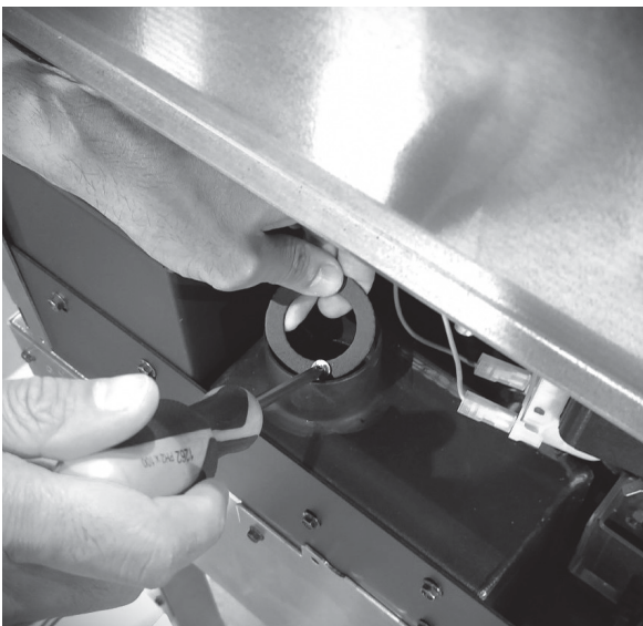
Fig. 88 - Retirer l'anneau
