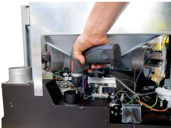
Fig. 41 - Extraction anneau 1
