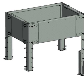
Fig. 44 - Assembler les jambes + la rallonge
