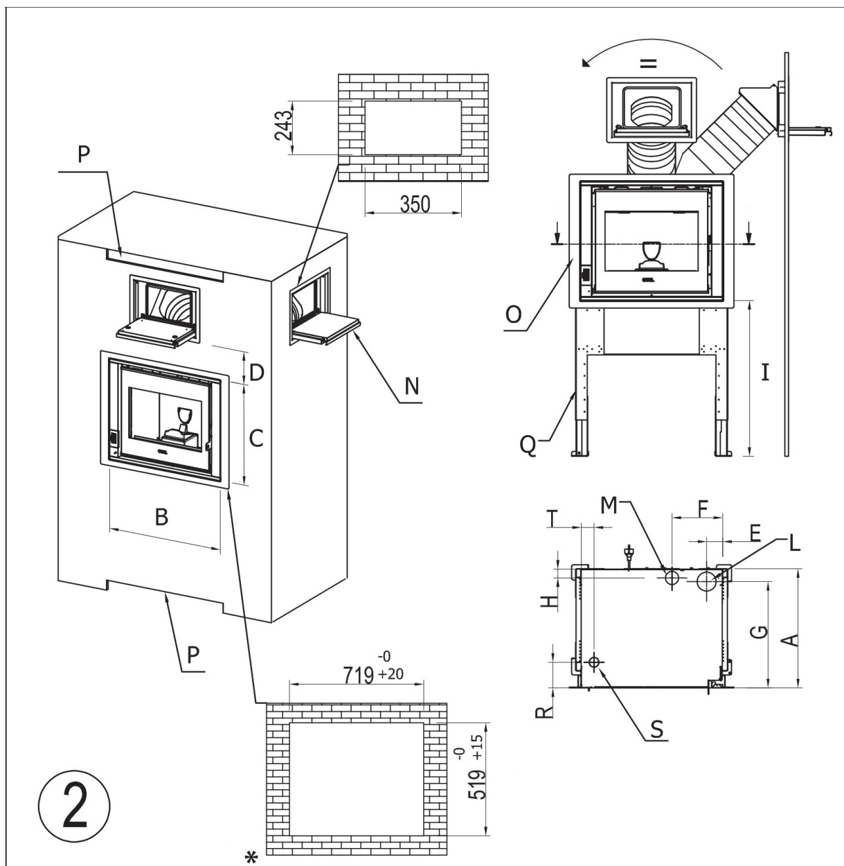
Fig. 24 - ZEN - ZEFIRO avec trappe + cadre
