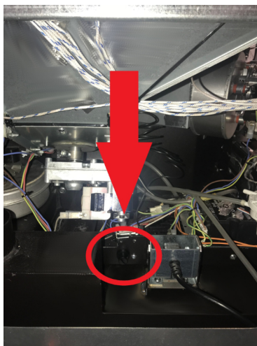
Fig. 43 - Réarmement manuel: il se trouve derrière le réservoir, près de la prise d'alimentation
