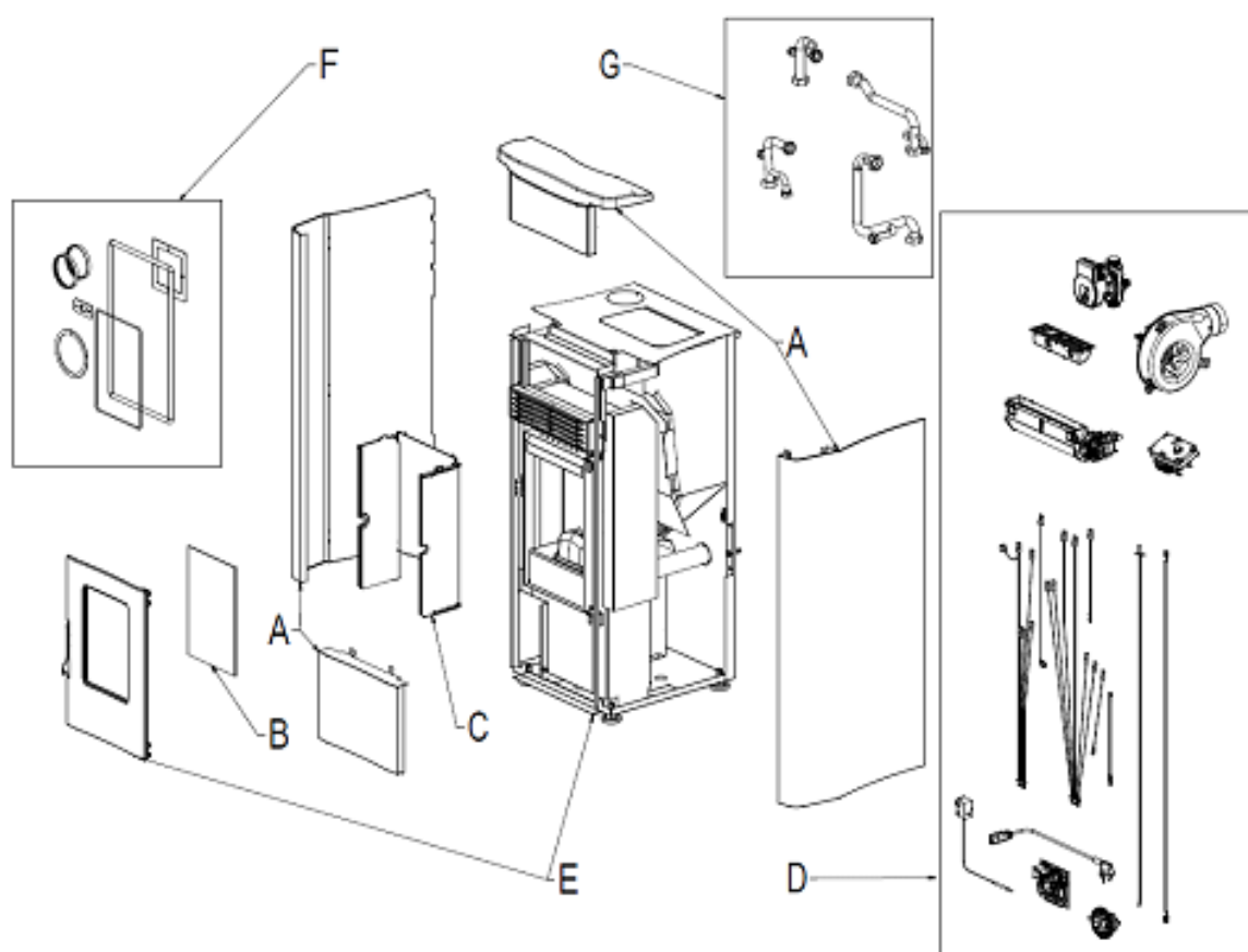
Fig. 1 - Dessin éclaté
