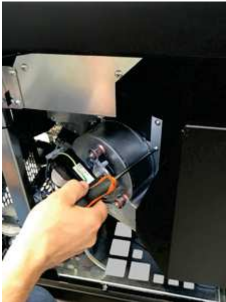
Fig. 36 - Retirer les vis
