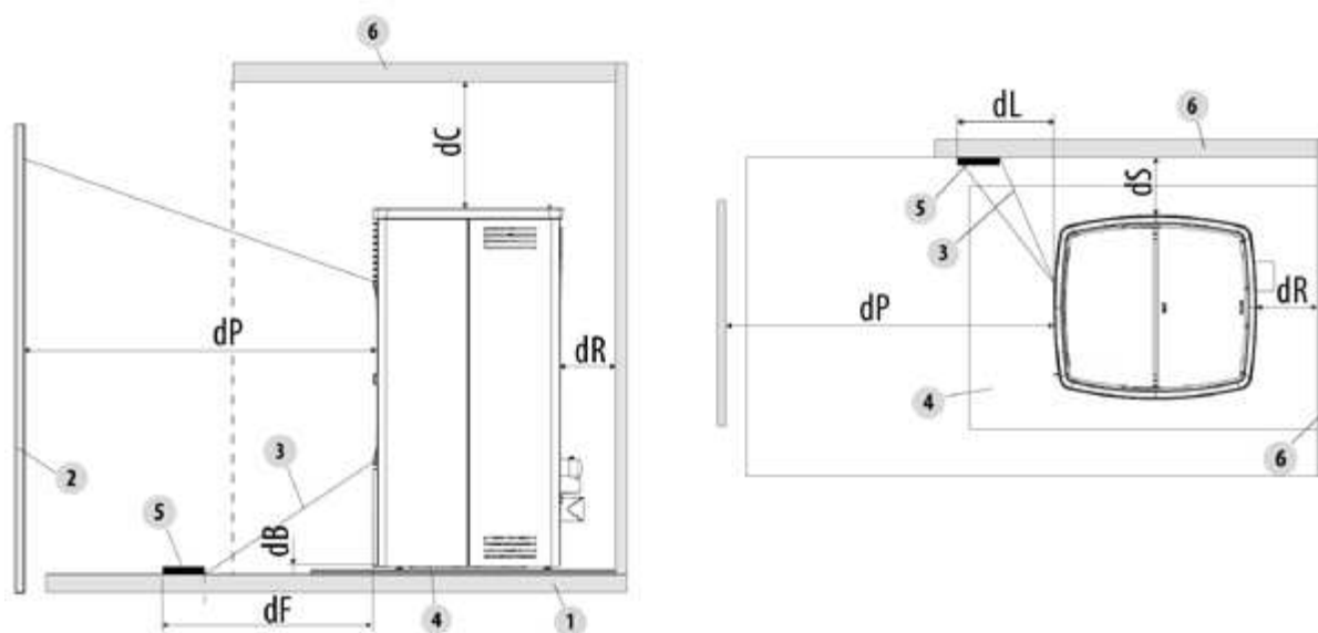
Fig. 20 - Distances de sécurité
