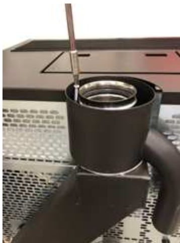
Fig. 51 - Fixer le concentrique sur le tuyau
