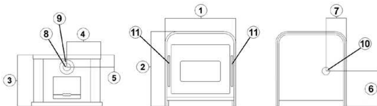
Fig. 22 - Dimensions générales: FRAME³ UP
