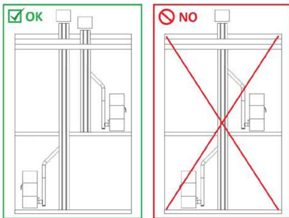
Fig. 4 - Exemples des installations correctes
