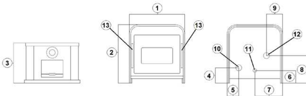
Fig. 21 - Dimensions générales: FRAME³
