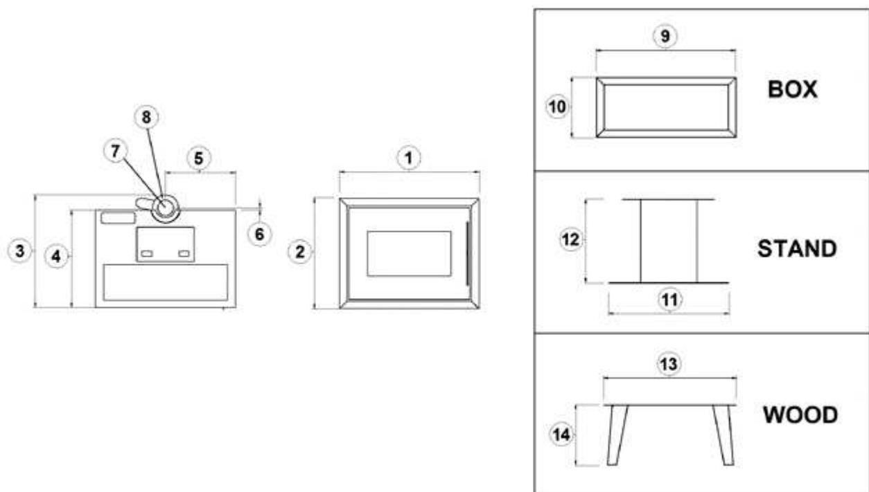
Fig. 24 - Dimensions générales: MODO AT
