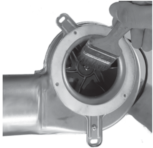
Fig. 71 - Nettoyage 2
