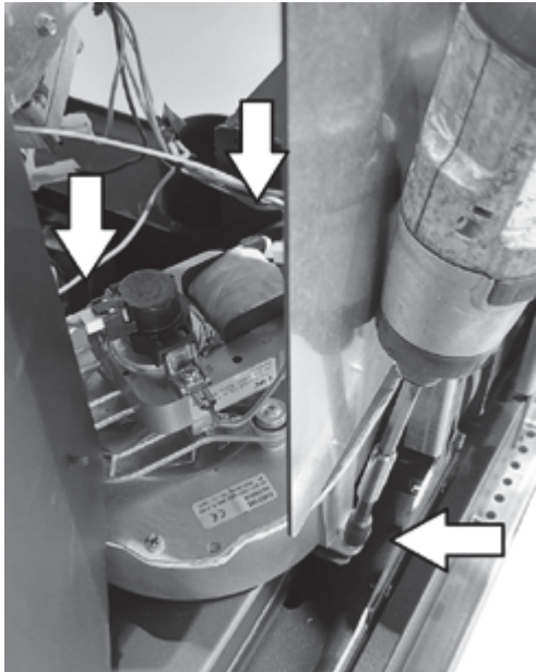
Fig. 70 - Retirer les vis - Nettoyage 1
