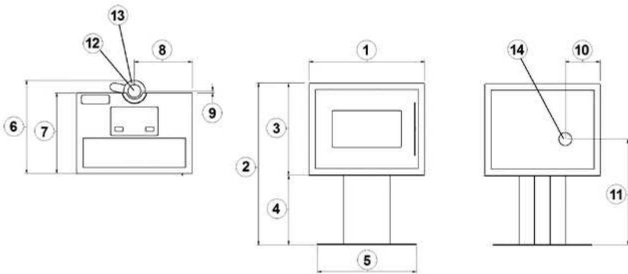
Fig. 23 - Dimensions générales: QUASIMODO³ UP
