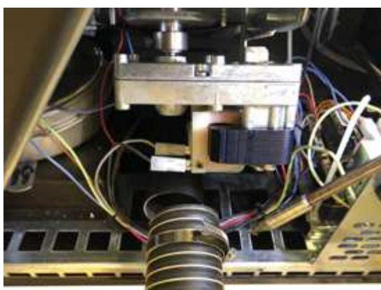
Fig. 53 - Branchement 2 entrées
