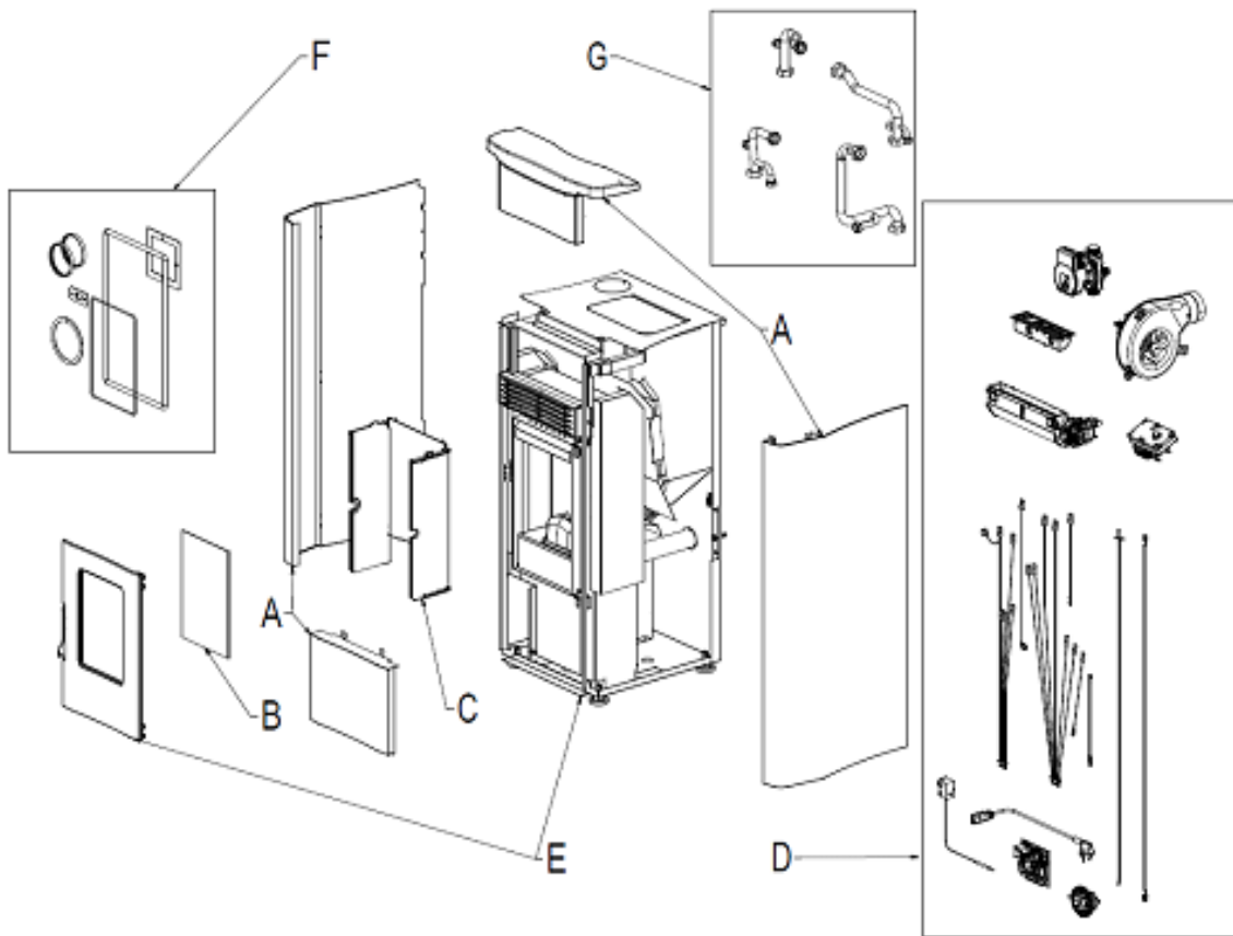
Fig. 1 - Dessin éclaté
