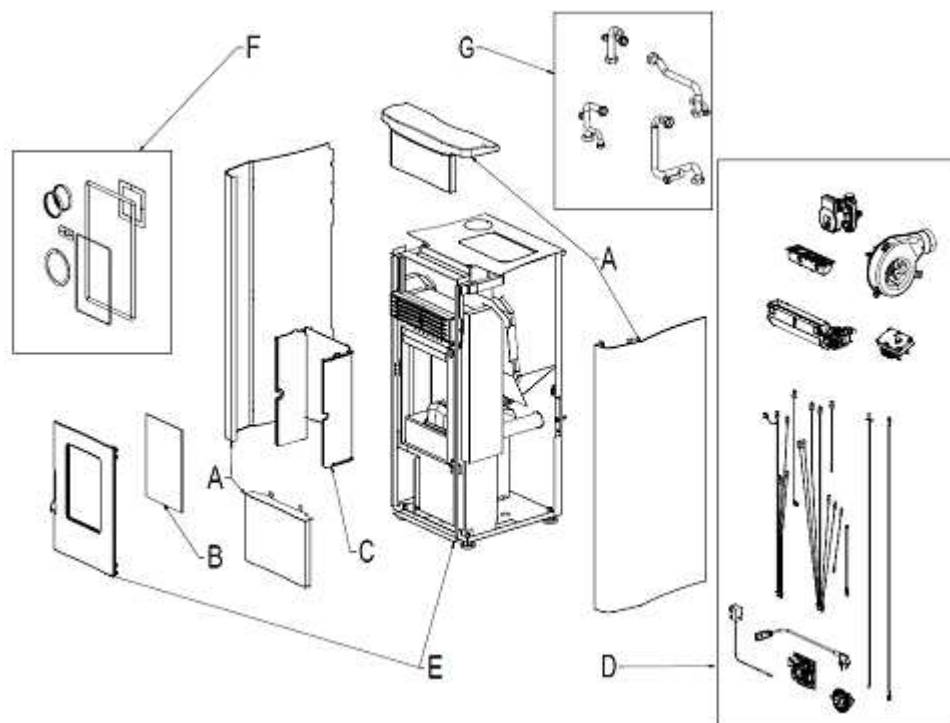
Fig. 1 - Dessin éclaté
