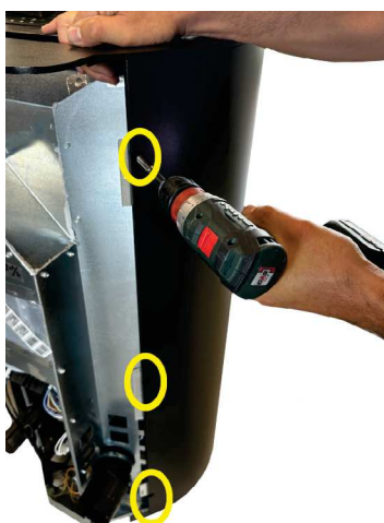
Fig. 32 - Retirer les vis.
