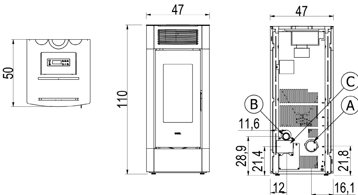
Fig. 26 - CRISTAL PLUS 9 T2
