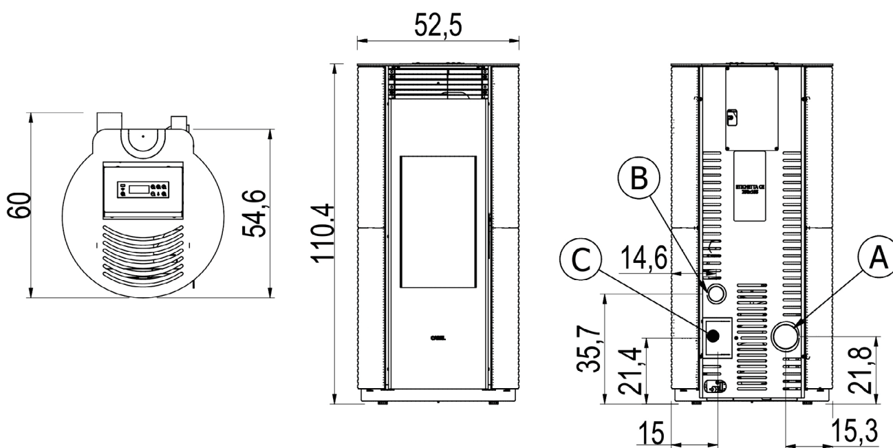
Fig. 22 - SPIN PLUS 9 T1
