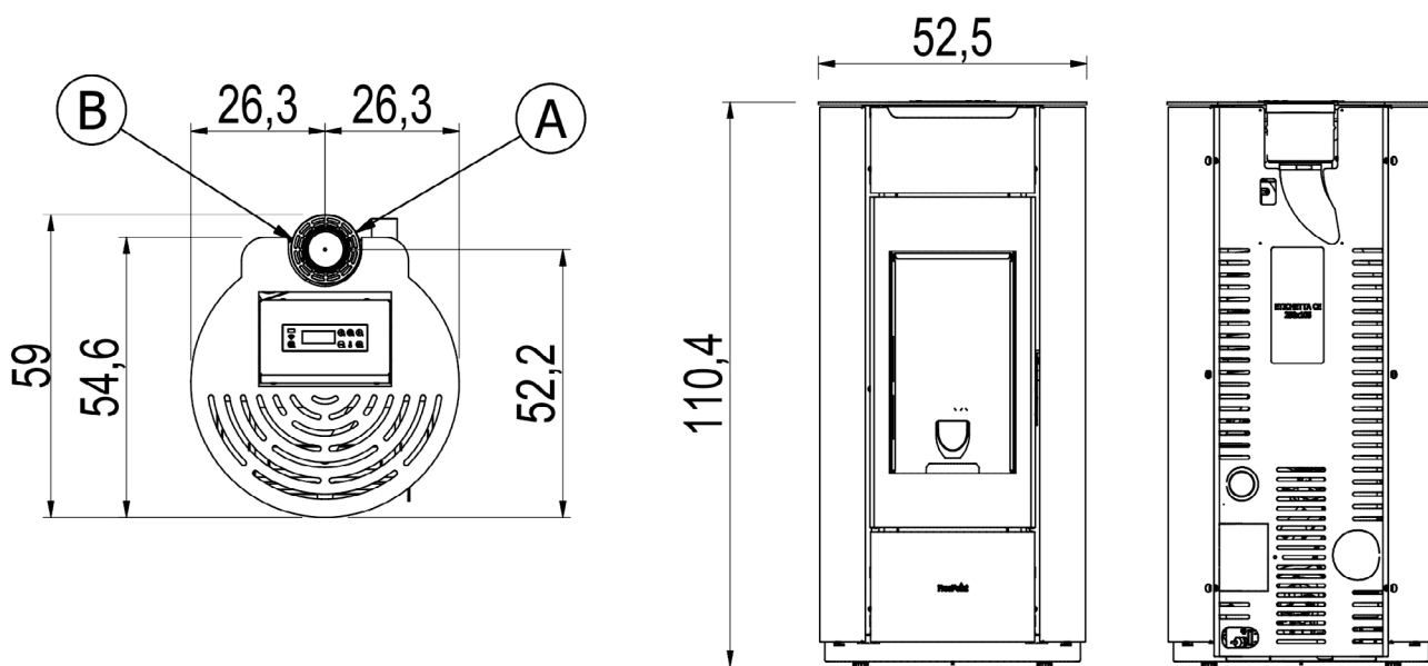
Fig. 24 - EOS 6 BI-FLUX T1 - EOS 8 BI-FLUX T1
