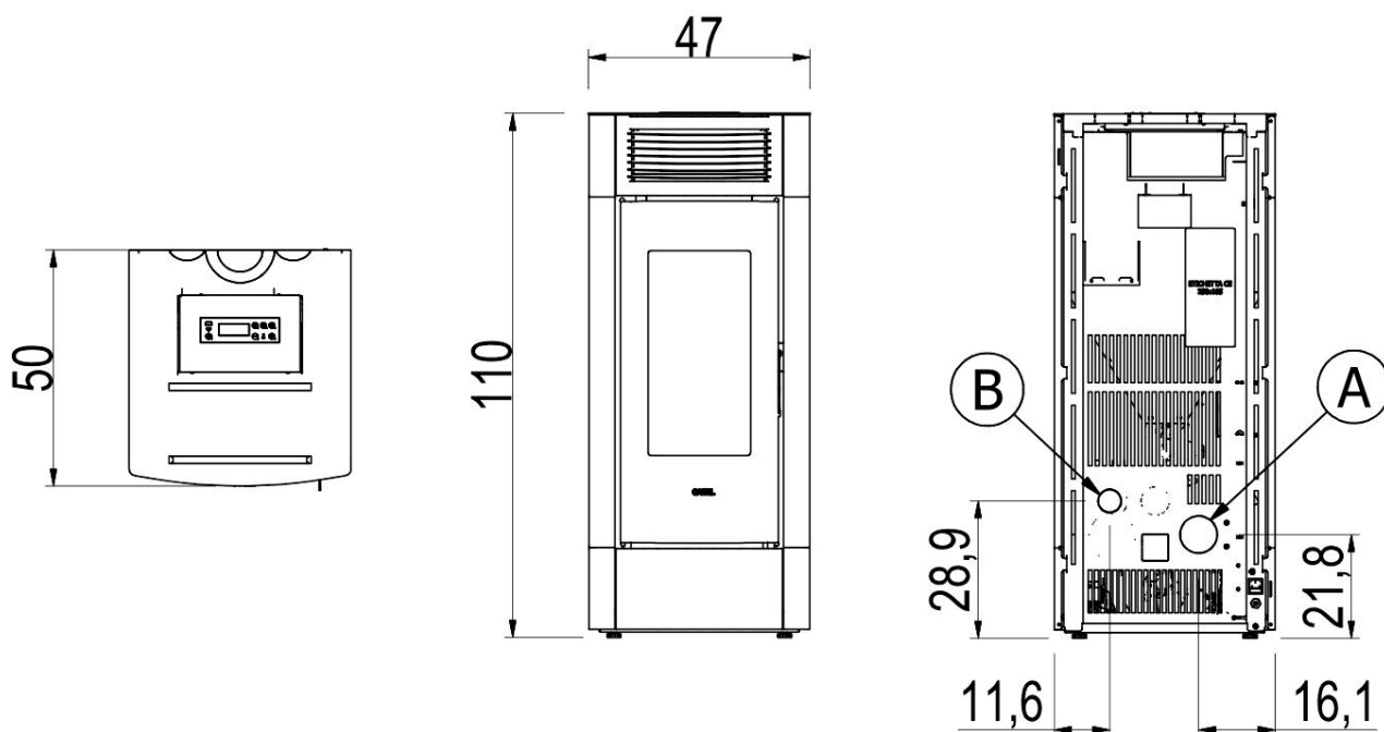
Fig. 25 - CRISTAL 9 AIR T1 - CRISTAL 9 AIRTECH T1
