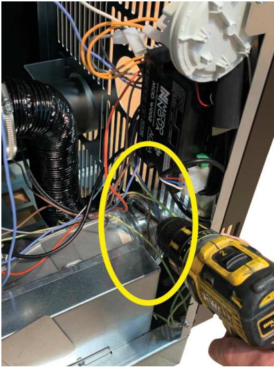
Fig. 59 - Extraire le tuyau flexible
