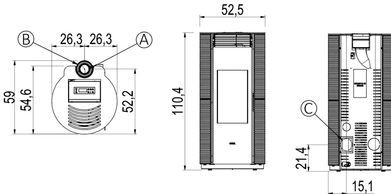
Fig. 21 - SPIN PLUS 9 UP-TWIN T1
