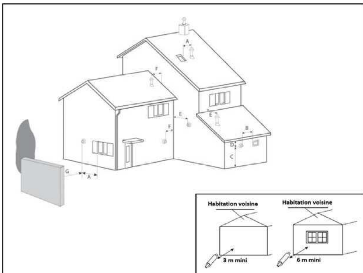
Fig. 15 - Position des terminaux
