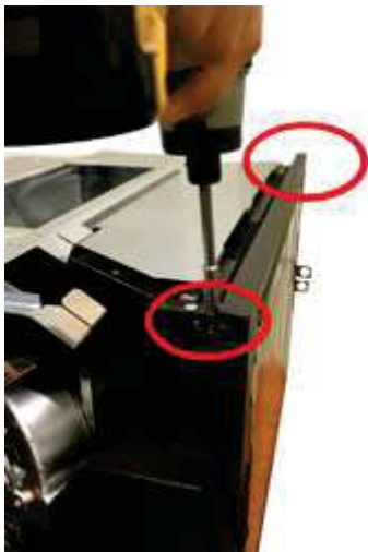
Fig. 62 - Retrait du profil supérieur
