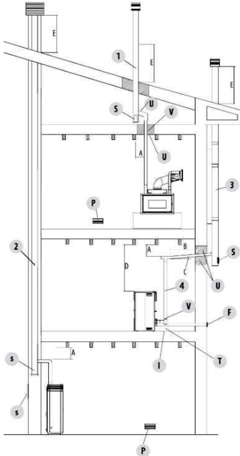
Fig. 13 - Conduit des fumées
