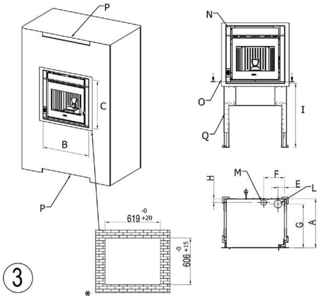
Fig. 25 - PONENTE - ZENITH tiroir + cadre
