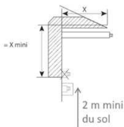
Fig. 16 - Rebord de toit
