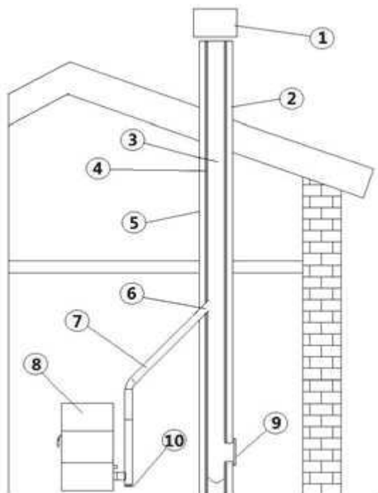
Fig. 2 - Composants de la cheminée
