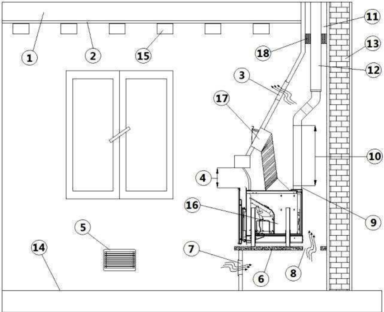
Fig. 35 - Installation sur la cheminée existante
