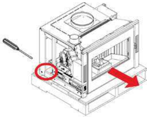
Fig. 1 - Retrait des vis
