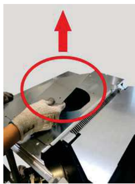
Fig. 75 - Retirer le bouchon
