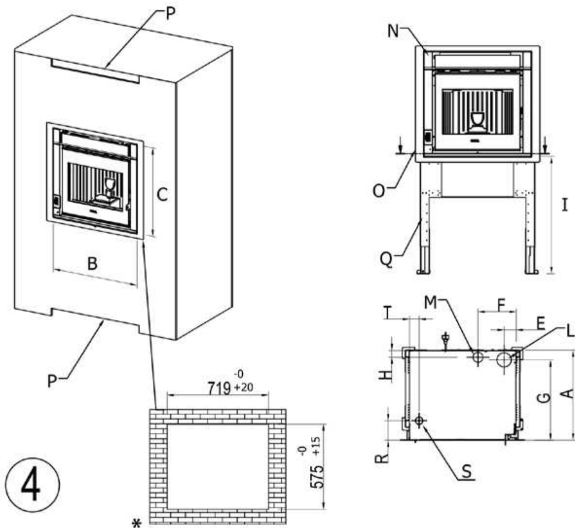
Fig. 26 - ZEFIRO-ZEN tiroir + cadre
