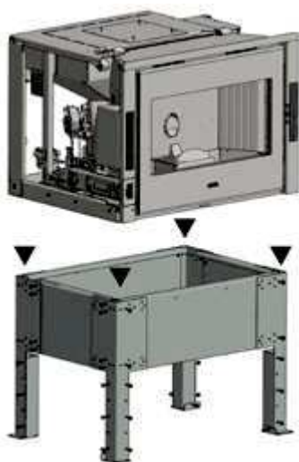
Fig. 45 - Fixer l'insert dessus
