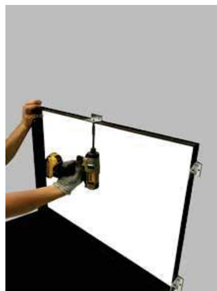
Fig. 87 - Fixation arrière 2
