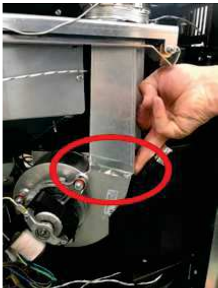
Fig. 56 - Sceller avec du ruban adhésif en aluminium
