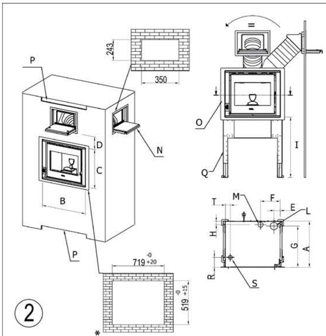
Fig. 24 - ZEN - ZEFIRO avec trappe + cadre
