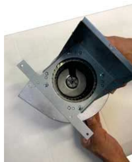
Fig. 52 - Tourner le ventilateur
