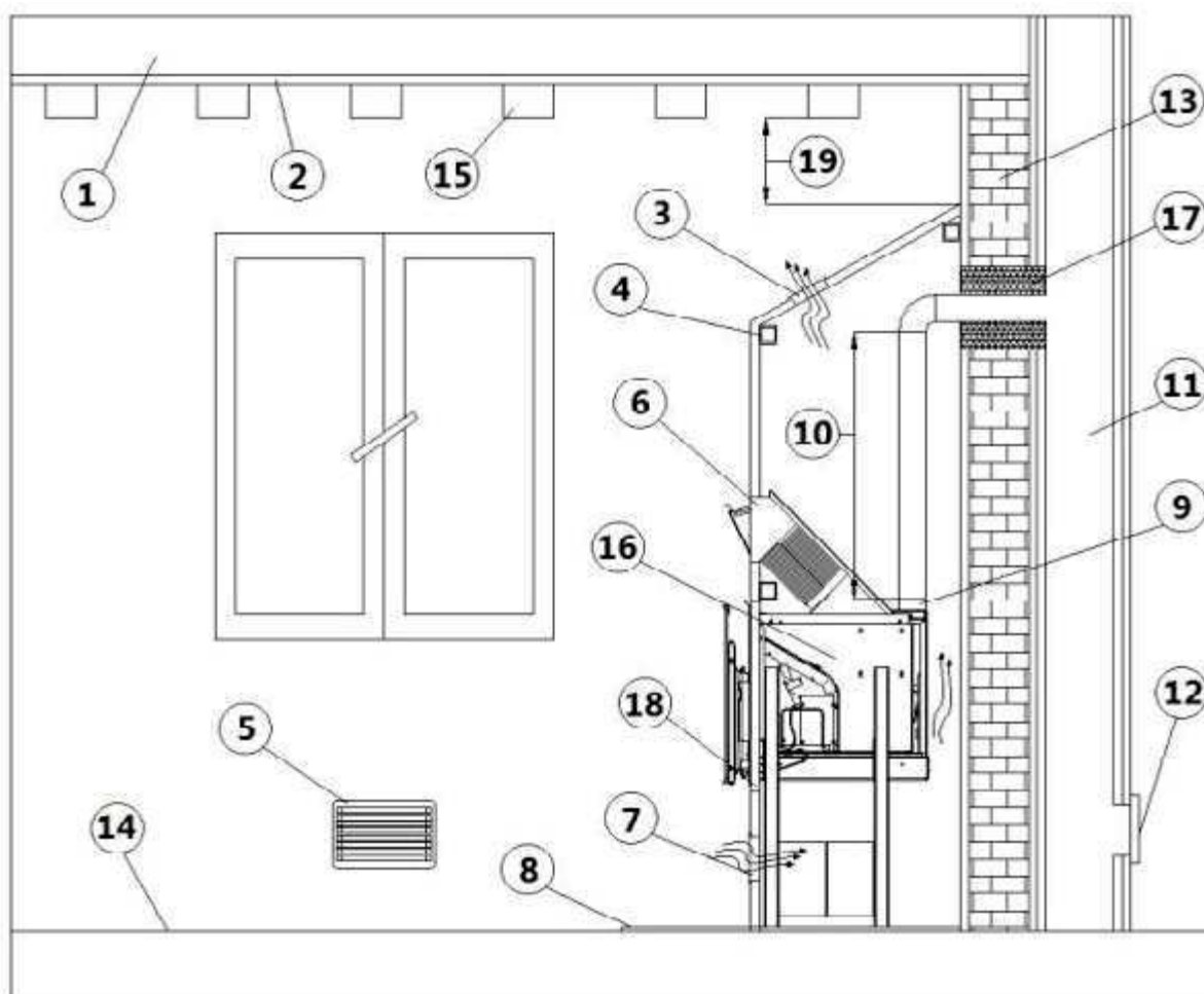
Fig. 34 - Installation avec le revêtement
