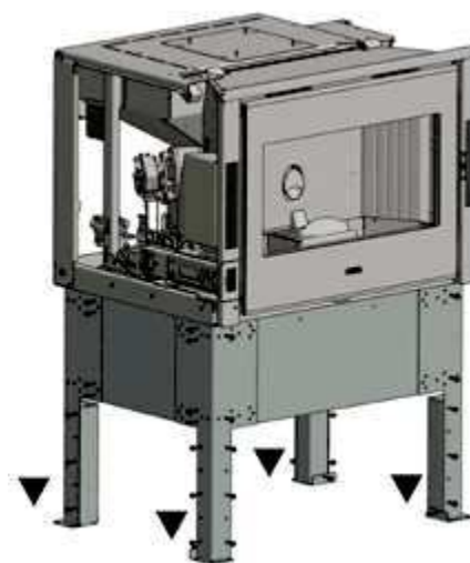
Fig. 46 - Fixer la structure au sol et au mur
