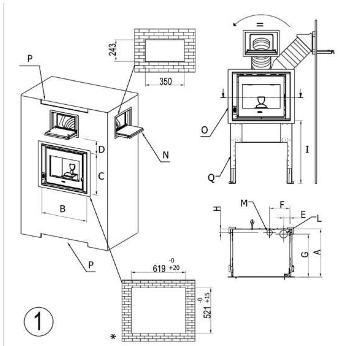
Fig. 23 - PONENTE - ZENITH avec trappe + cadre
