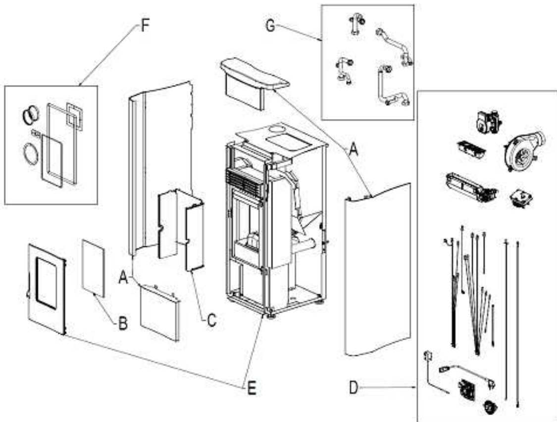
Fig. 1 - Dessin éclaté
